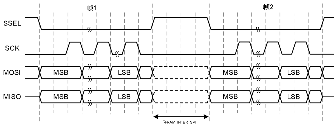
图3 SPI 帧间隔
