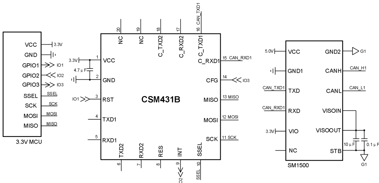
图 5 SPI 转 CANFD1 参考电路
