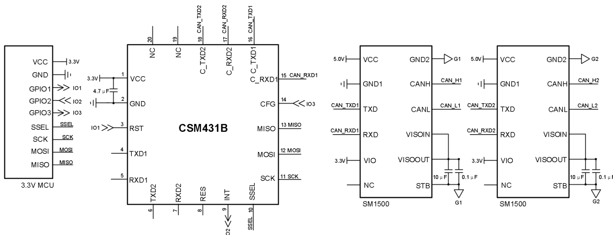
图 6 SPI 转 CANFD1 和 CANFD2 参考电路
