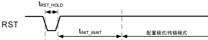
图 1 复位时序
