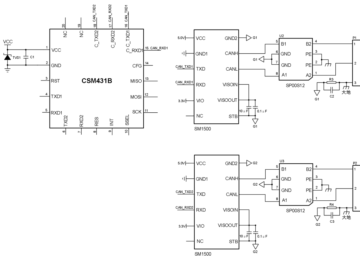
图 10 外围保护电路 1
