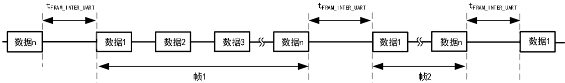
图 2 UART 帧间隔
