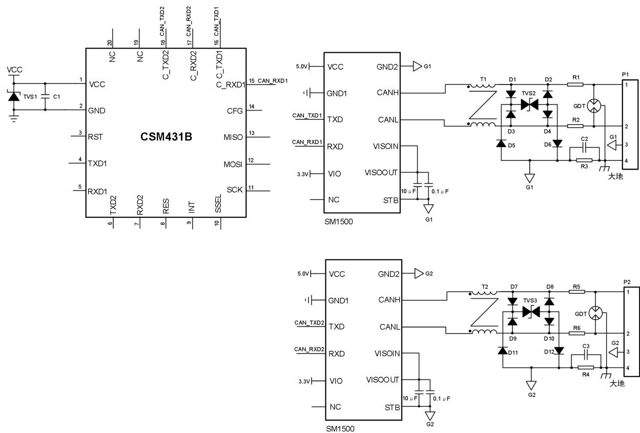
图 11 外围保护电路 2
