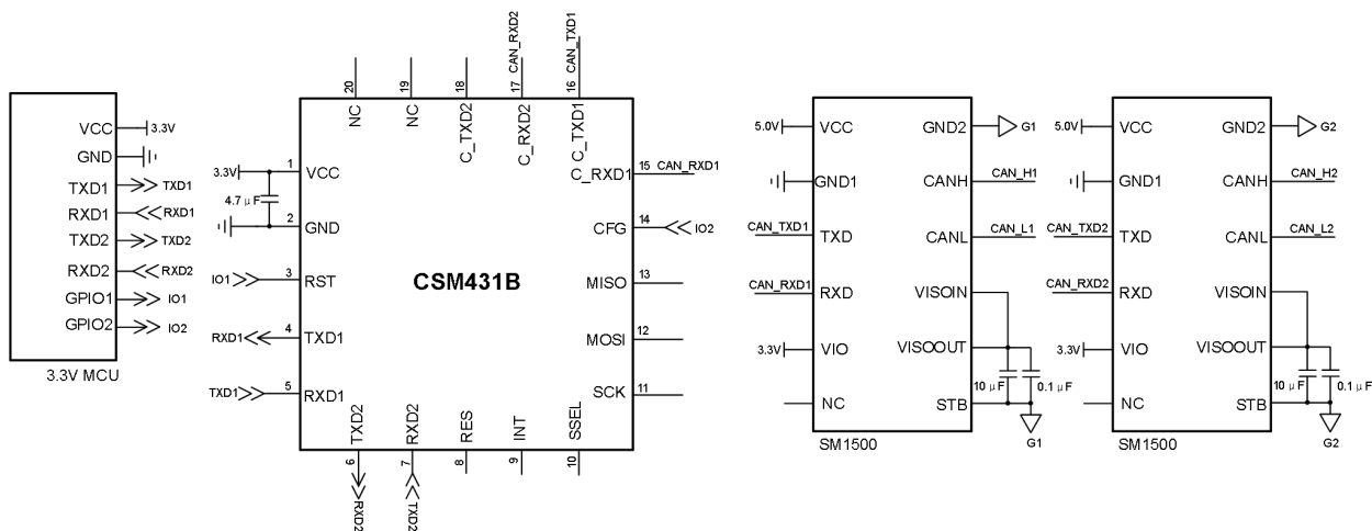
图 9 UART1 和 UART2 转 CANFD1 和 CANFD2 参考电路
